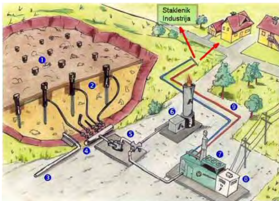
Слика 95 - Шематски приказ експлоатације депонијског гаса у циљу добијања енергије
